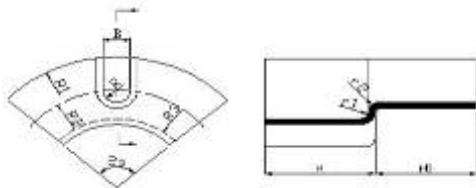
A、U形槽保护正角环片 U-shape Snout Angle Cap
